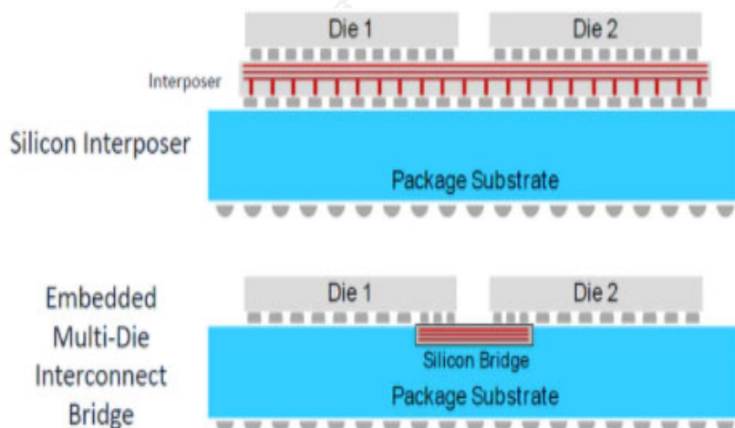
圖二、2.5D 封裝示意圖
