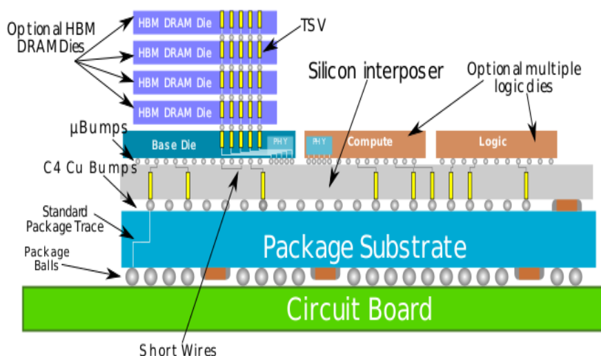
圖三、3D 封裝示意圖
